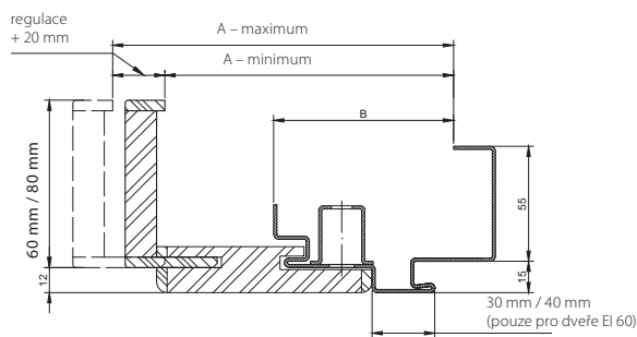
průřez zárubně PROJEKT
